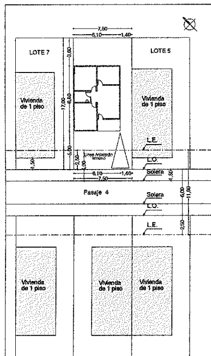
Emplazamiento Escala 1:500
